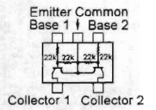
UMC5N (C5) (Q1008, 1031)
