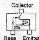
DTC124EE (2E) (Q1001, 1004, 1048)
