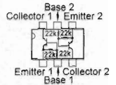
UMD2N (D2) (Q2012, 2013, 2025)
