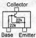
DTA124EE (15) (Q1027)
