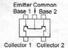
UMW1 (W1) (Q1019, 1021) XP1501 (5R) (Q1037)
