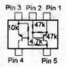
UMC5N (C5) (Q1008, 1031)
