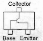
2SC4537 (IS-) (Q1007, 1032) 2SC4226 (R22) (Q1022, 1023, 1042) 2SC4227 (R32) (Q1043, 1044) 2SC4245 (HB) (Q1030) 2SC4116GR (LG) (Q1038) 2SC4215Y (QY) (Q1041) 2SC4228 (R42) (Q1045, 1046)
