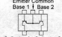
FMW1 (W1) (Q2006)
