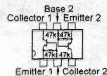
XP4213 (8S) (Q1013, 1015)
