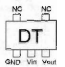
S-80730SN (DT) (Q2003)
