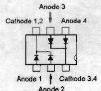
UMN11N (N11) (D1027)
