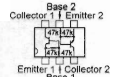
XP4213 (8S) (Q1028)
