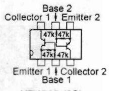
XP4213 (8S) (Q1028)
