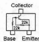
DTC124EE (25) (Q1009, 1010)
