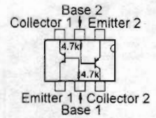
UMB3N (B3) (Q1029)
