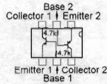
UMB3N (B3) (Q1029)
