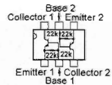
UMD2N (D2) (Q1002)
