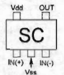
TC75S51F(SC) (Q1025)
