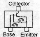
DTA144EU (16) (Q2017)
